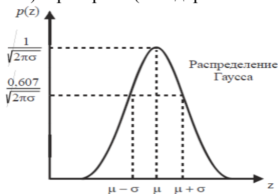
Рис. 1. Распределение Гаусса
